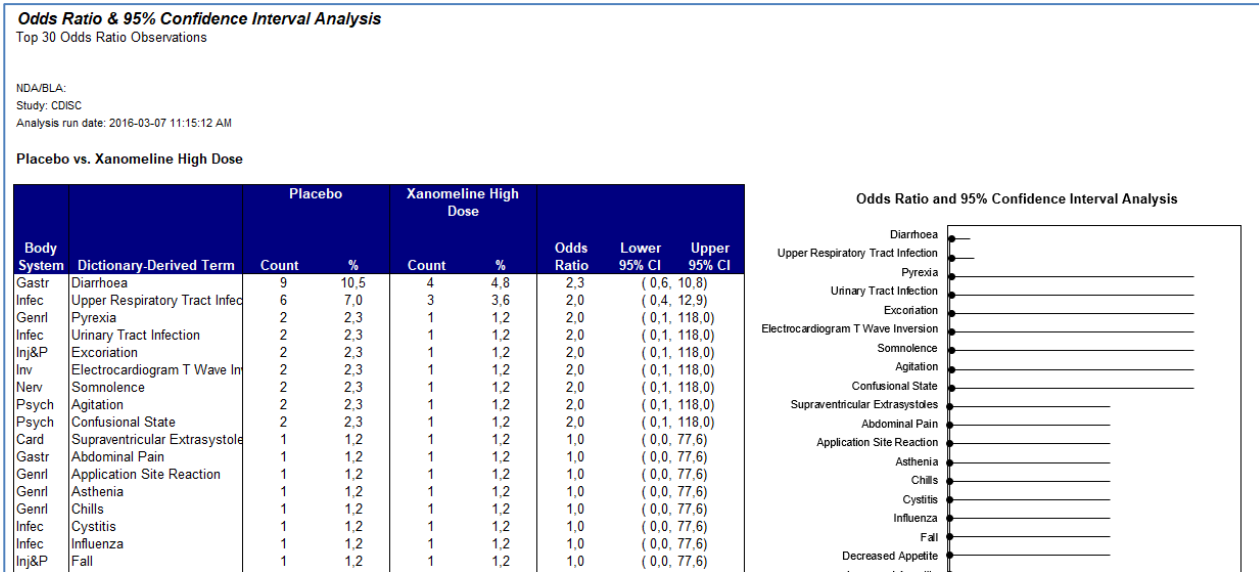
Abbildung 6: Beispielausgabe zu Konfidenzintervallen
