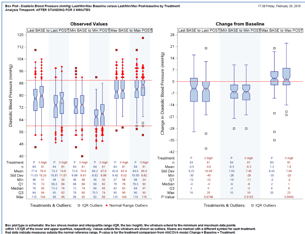
Abbildung 3: BoxPlot Beispiel
