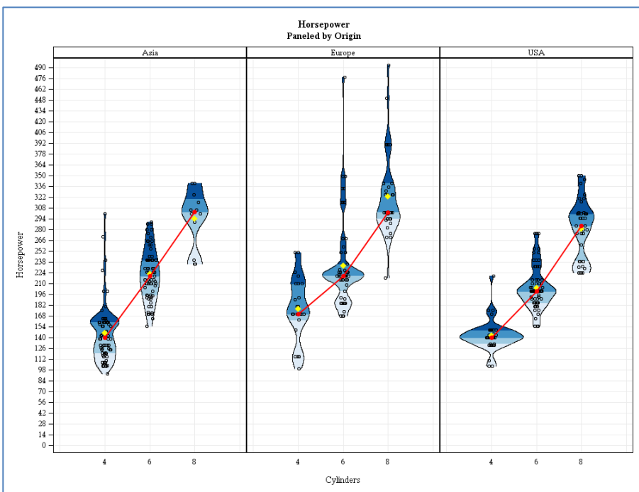
Abbildung 9: Beispiel eines Violin-Plots
