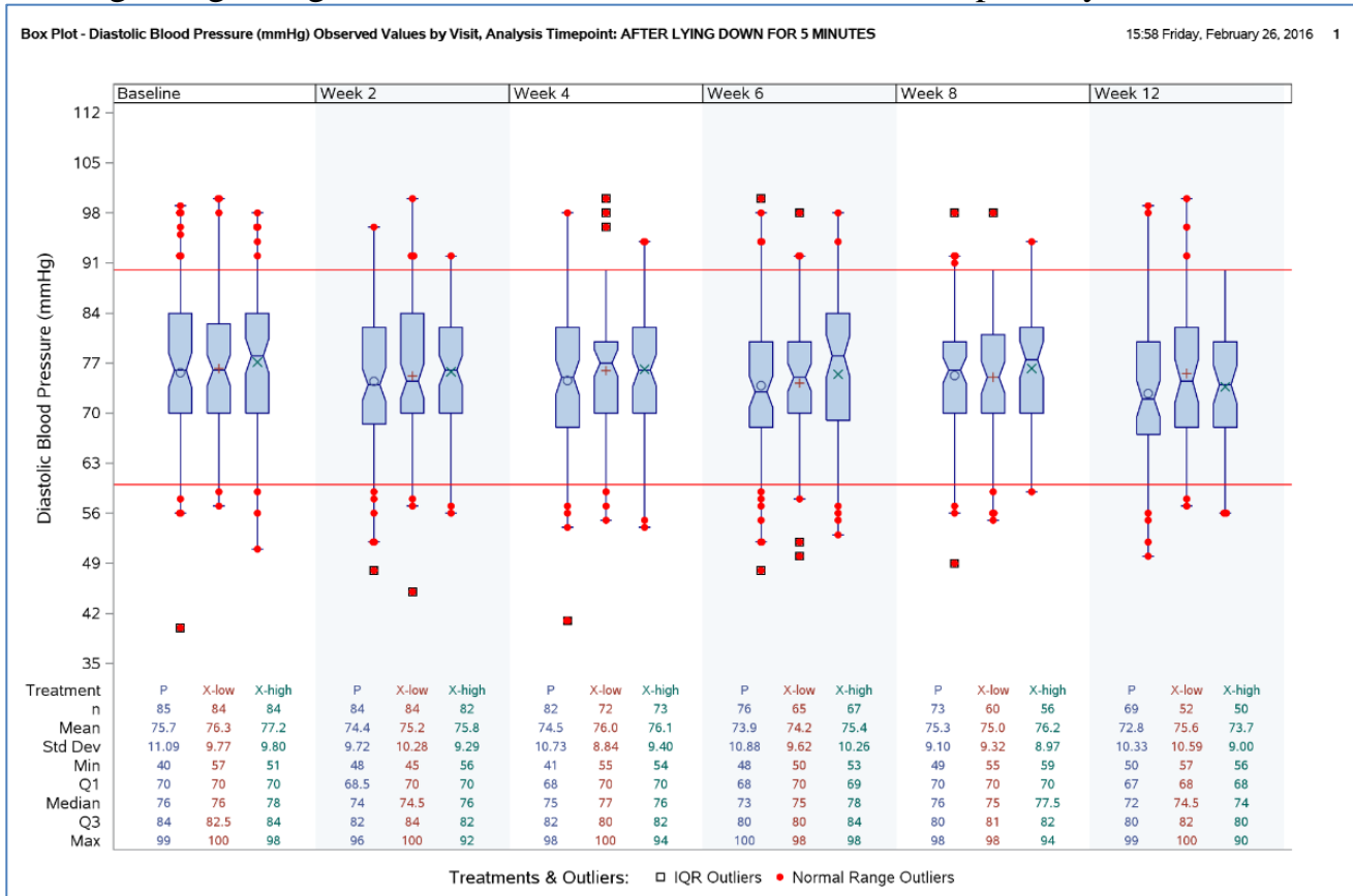
Abbildung 2: BoxPlot als Anwendungsbeispiel
