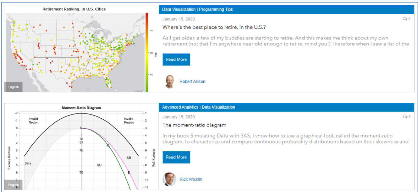
Abbildung 8: SAS Blogs
